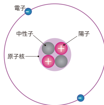
ヘリウム原子のモデル図
